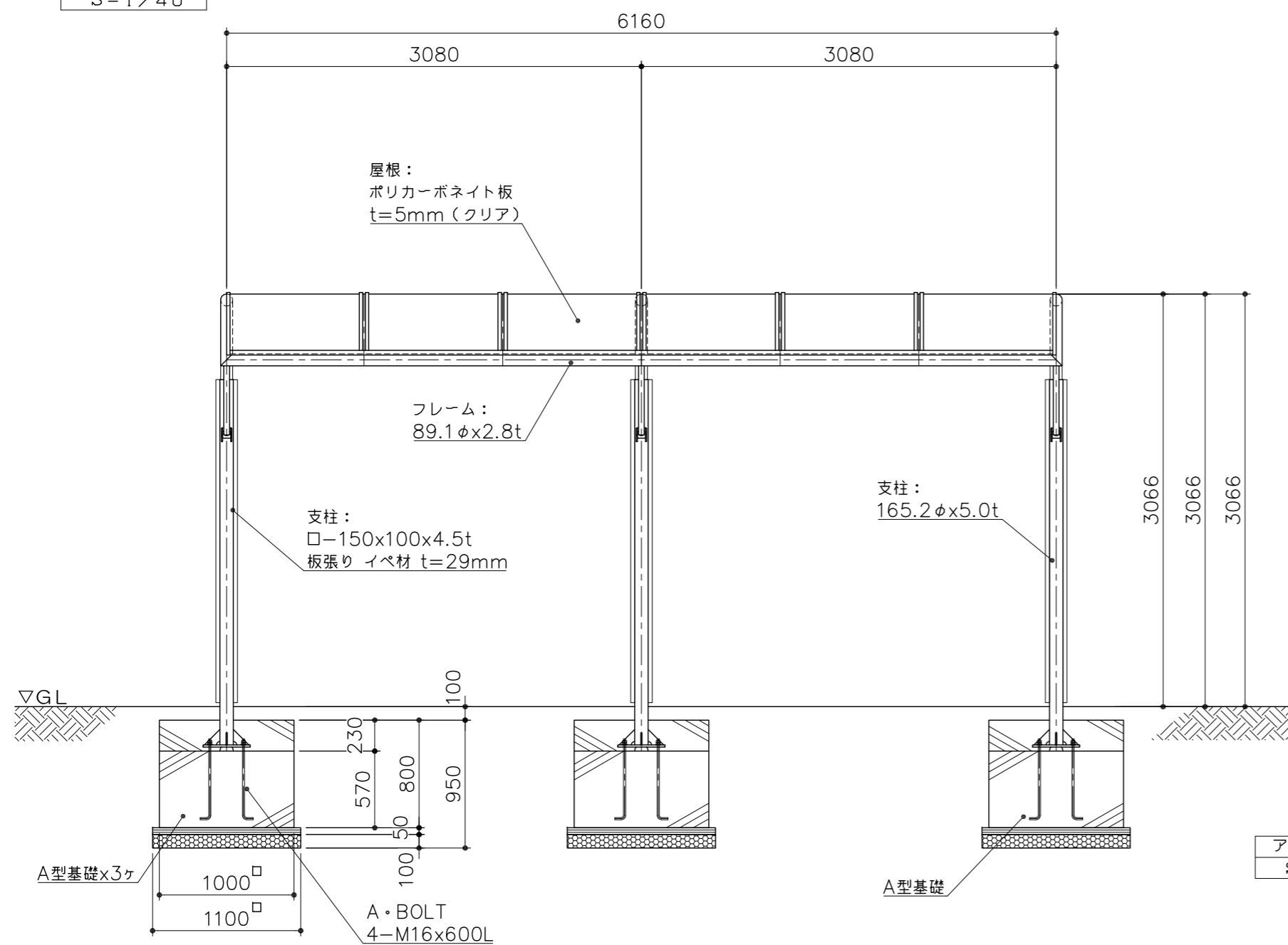
立面図 S = 1/40
