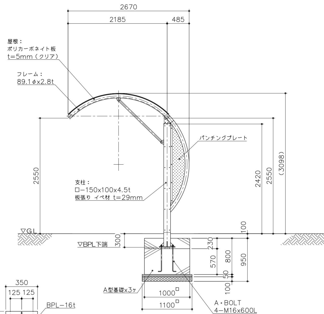
側面図 S = 1/40
