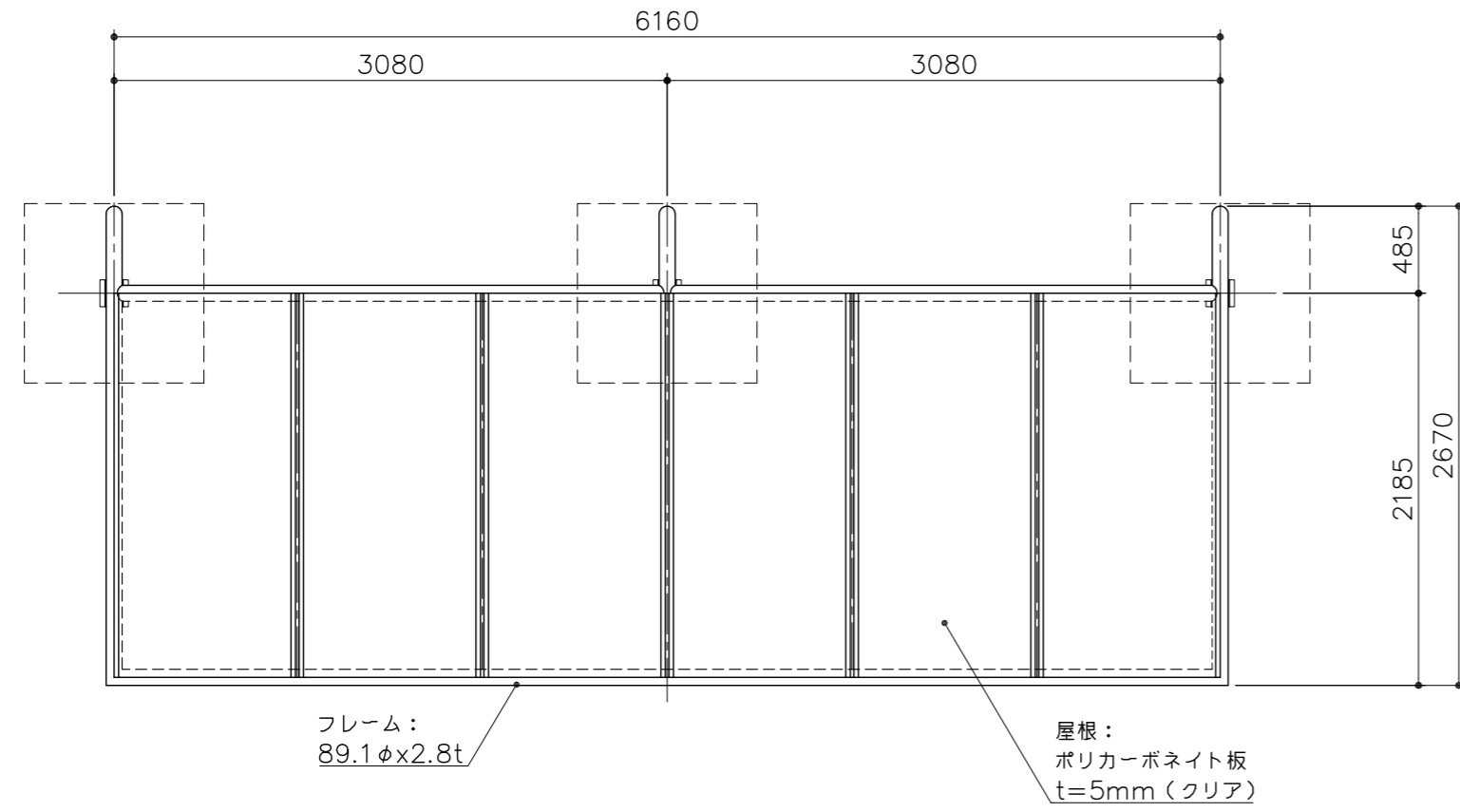
立面図 S = 1/40
