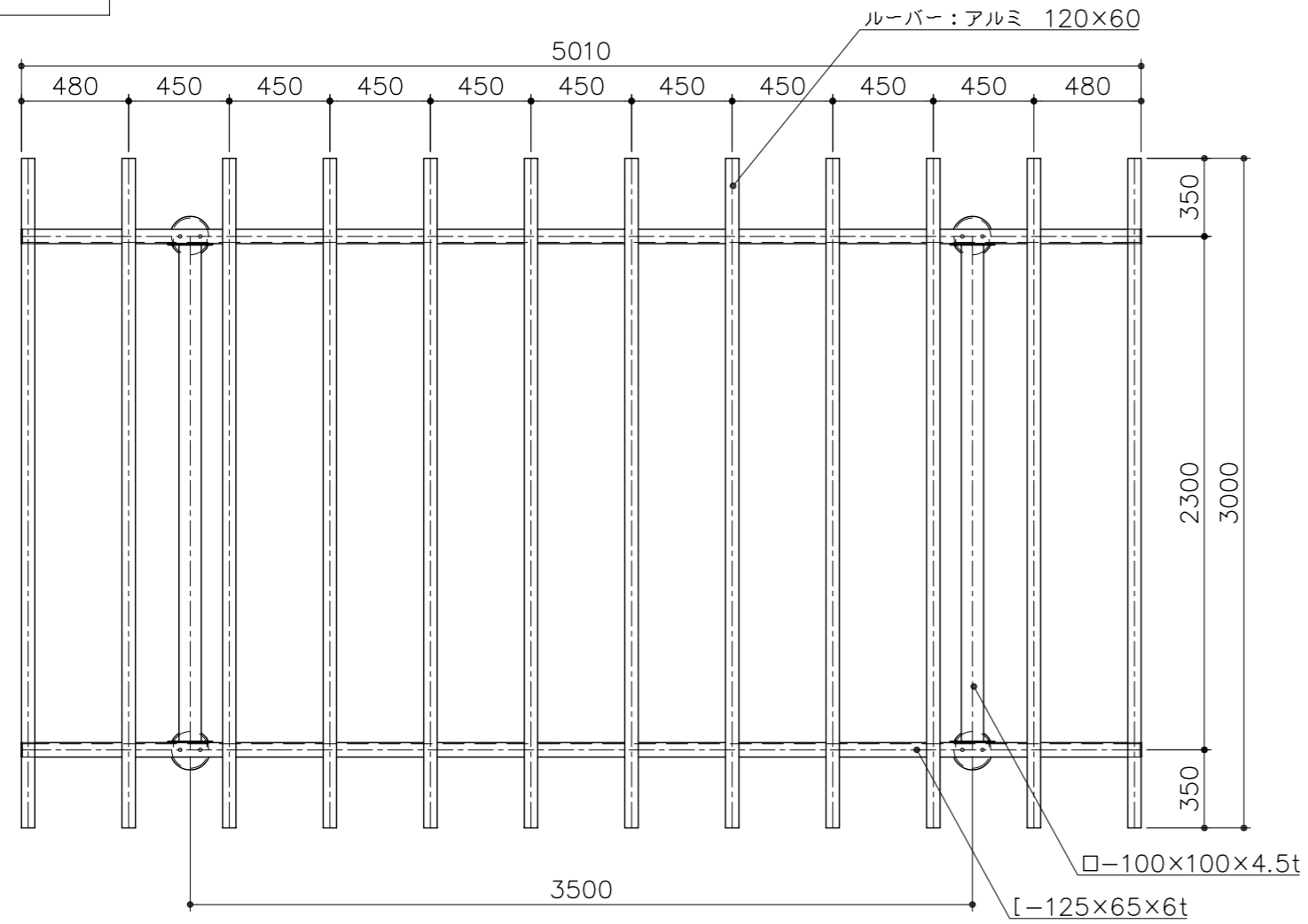
立面図 S= 1:30
