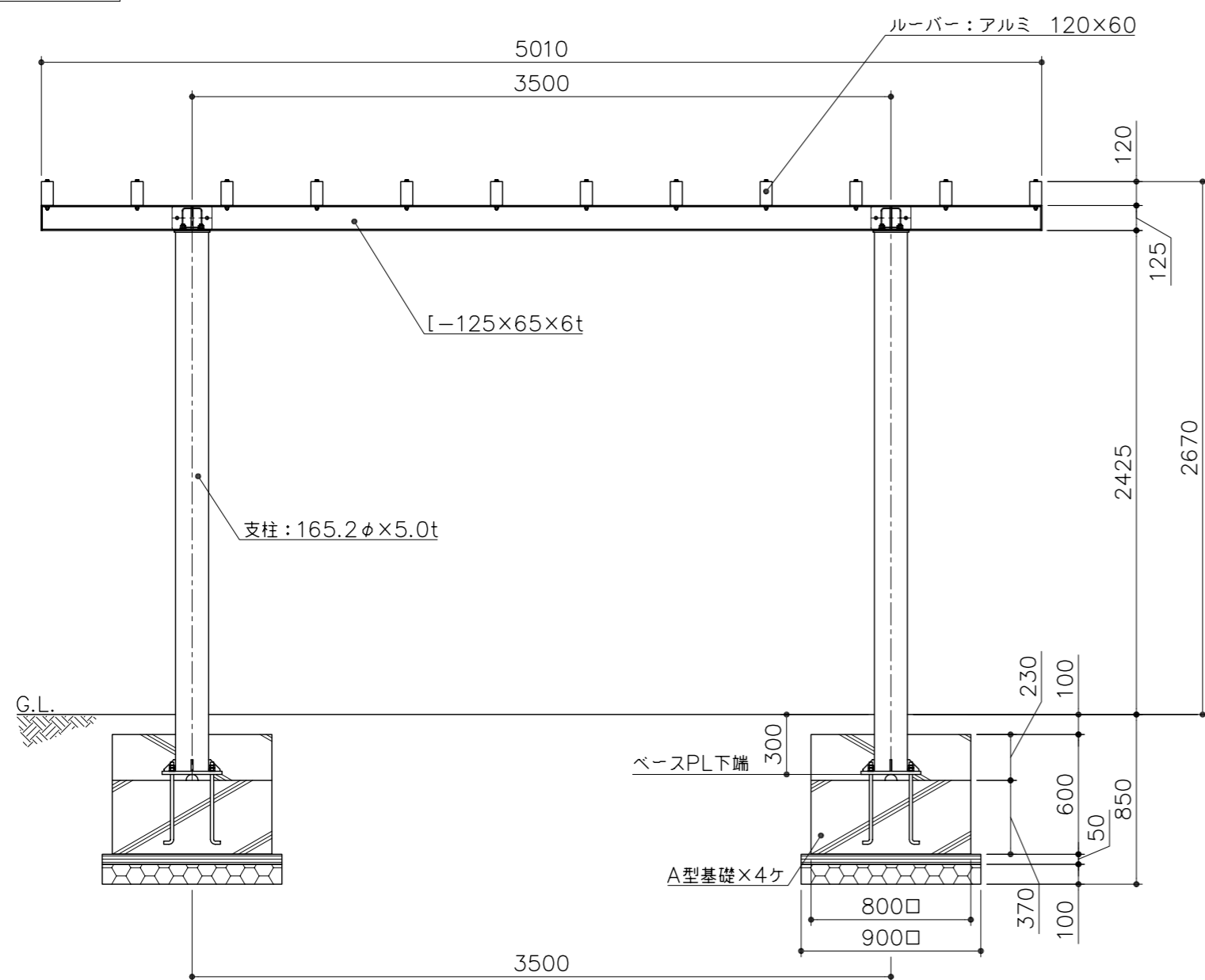
立面図 S= 1:30
