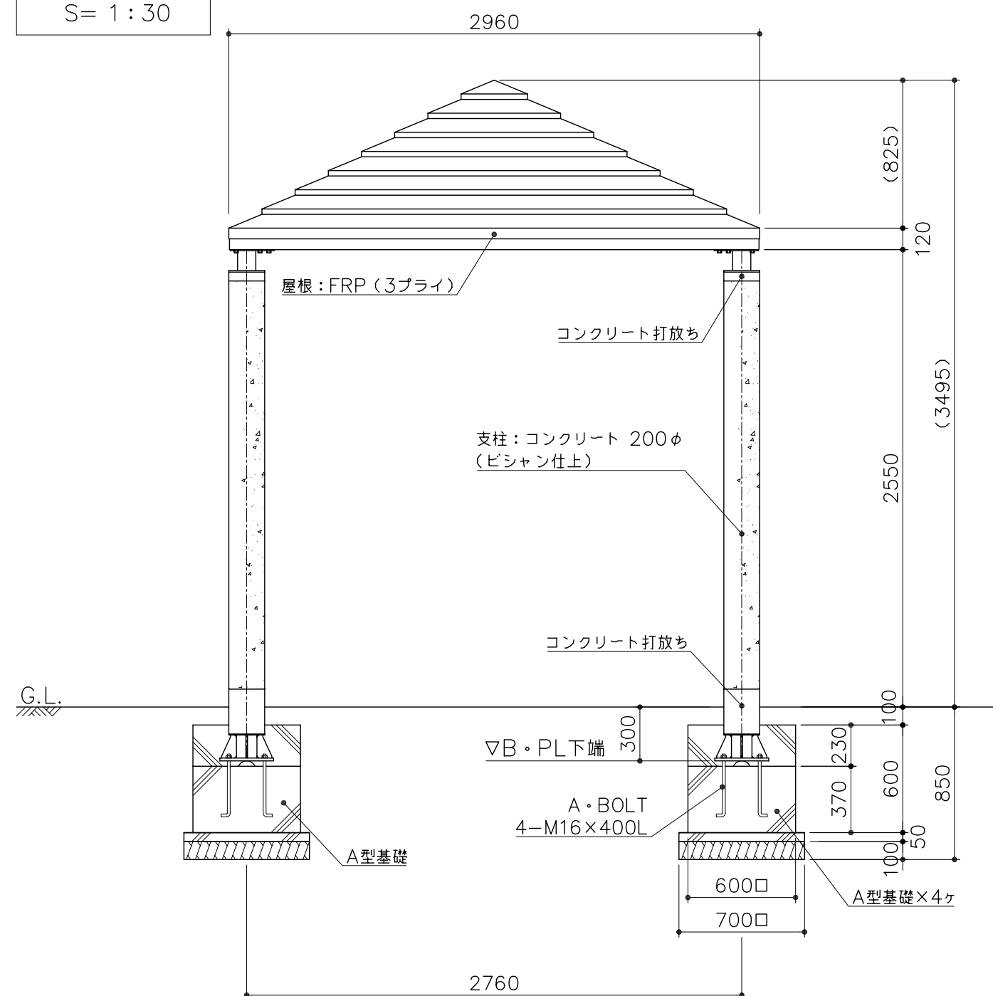
立面図 S = 1 : 30
