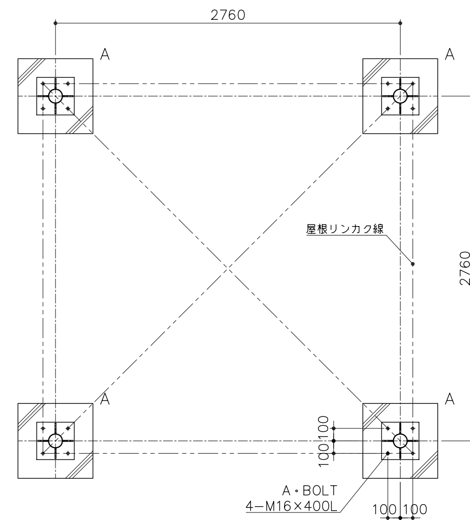
アンカープラン S = 1 : 10
