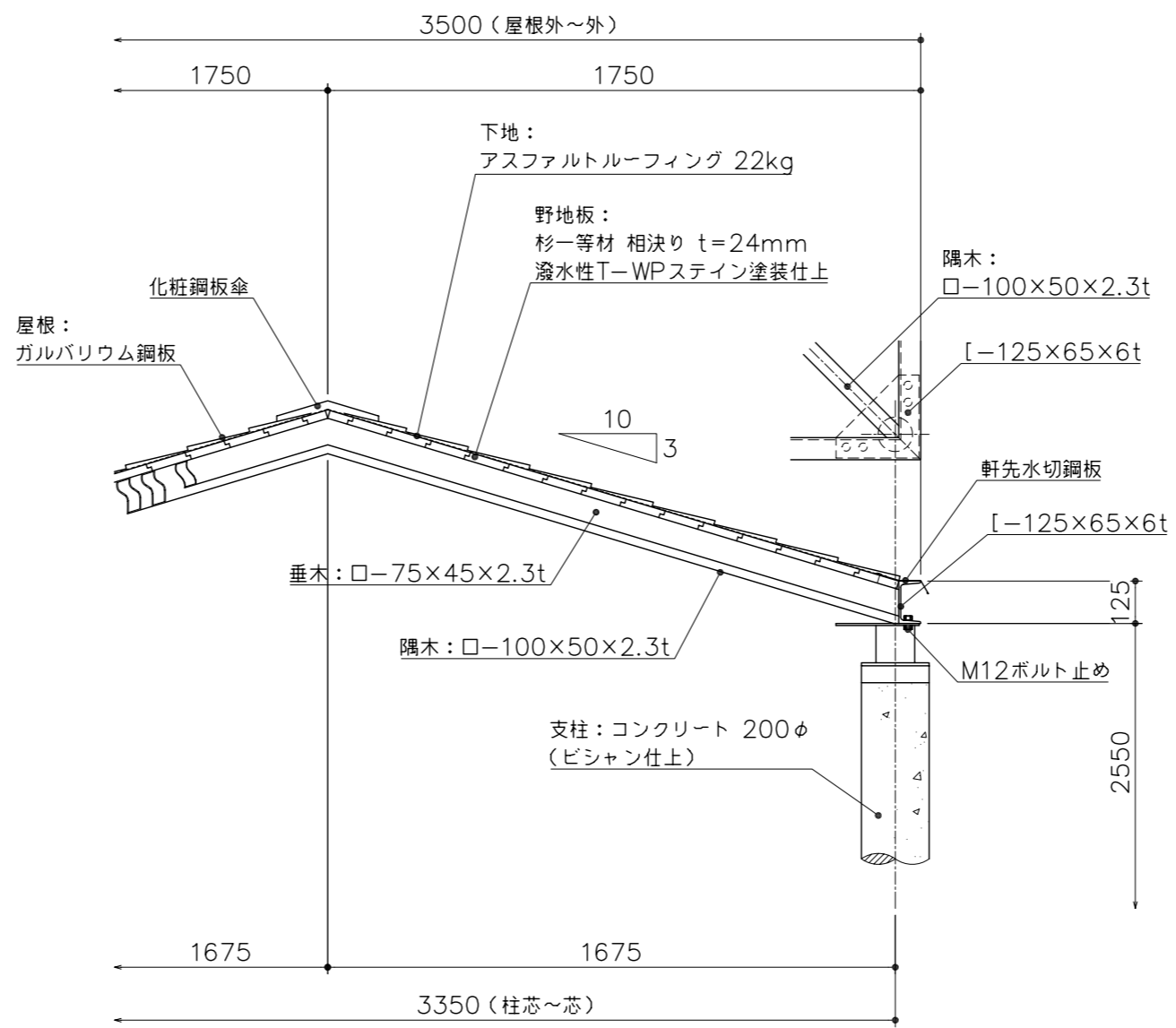
PG10-PS161 シェルター (PCコンクリート柱) S=図示 (BB)
