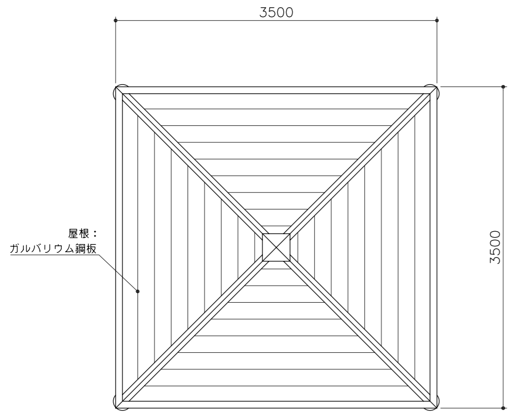
平面図 S= 1:40
