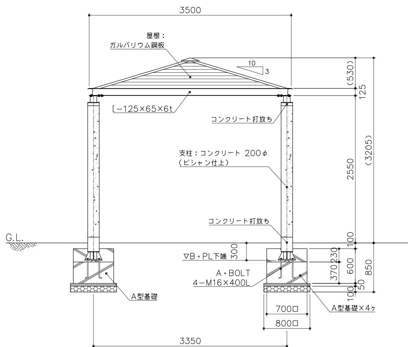
立面図 S= 1:40
