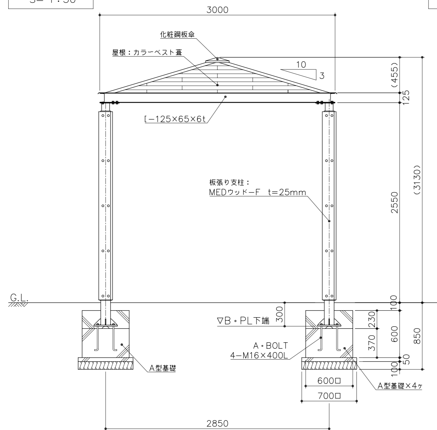
立面図 S= 1:30
