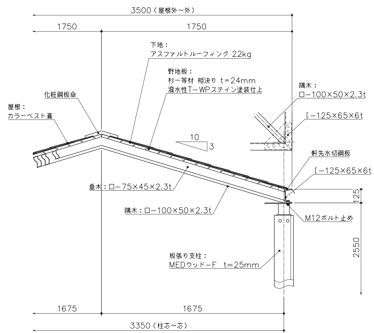
PG10-PS170 シェルター (リサイクルウッド柱) S= 図示 (BB)
