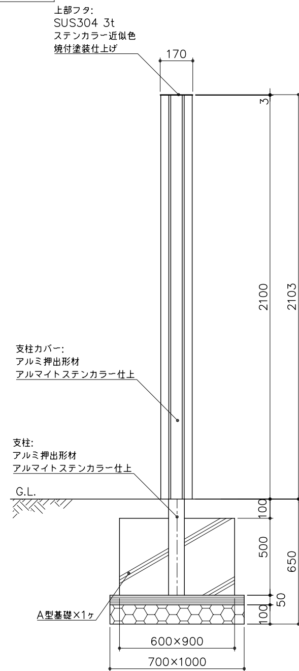
側面図 S= 1:20
