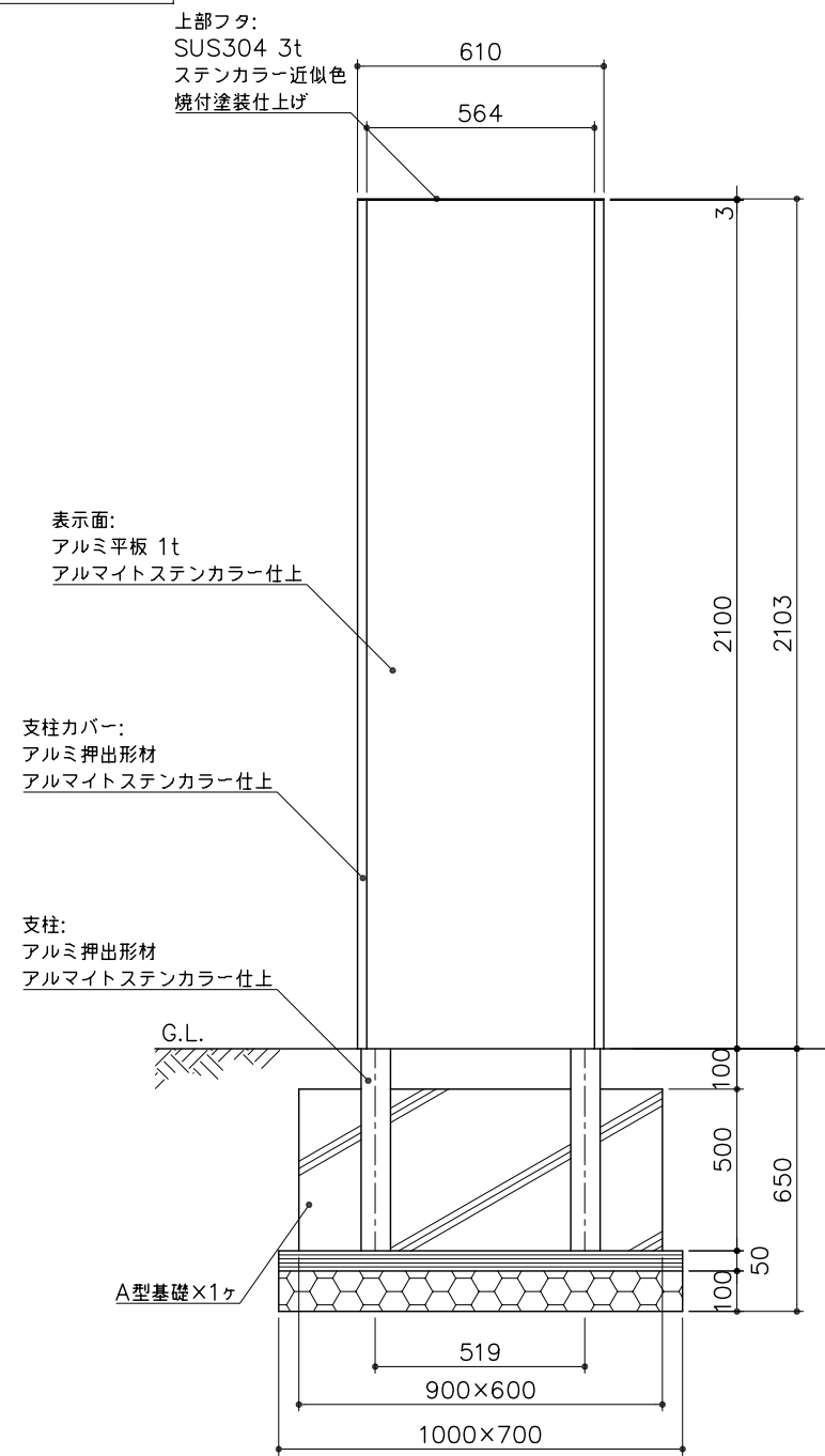
立面図 S= 1:20
