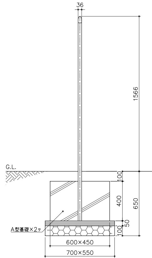
側面図 S= 1:20
